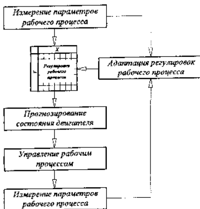
Рис. 8.3.2 Адаптация регуляторов рабочего процесса по результатам непосредственного измерения параметров управления.
