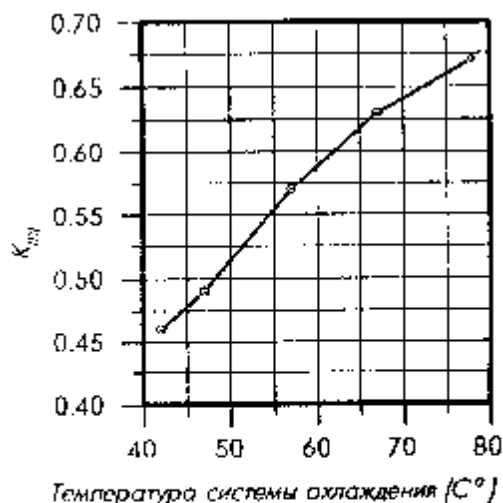
Рис. 4.1.5 Зависимость коэффициента использования топливоподачи от температуры охлаждающей жидкости в системе охлаждения. n=1200 \text{ мин}^{-1} , l = 1 \text{ см} , T_{\text{св}} = 160^\circ \text{C}
