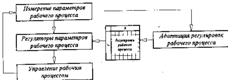
Рис. 8.3.1 Адаптация регуляторов рабочего процесса по результатам работы регуляторов параметров рабочего процесса двигателя.
