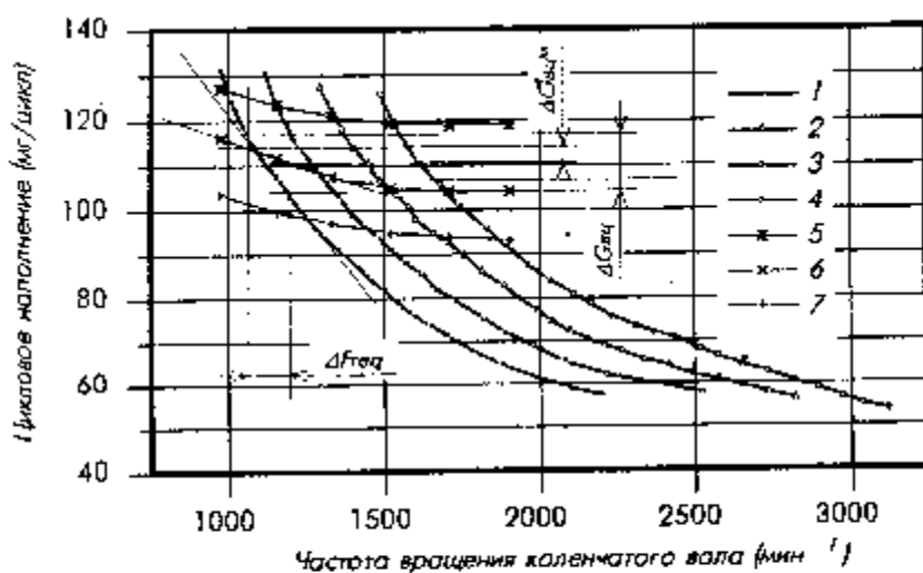
Рис. 7.3.3. Зависимость циклового наполнения двигателя от частоты вращения коленчатого вала двигателя при фиксированном положении РДВ (кривые 1-4) и при работе двигателя на холостом ходу с различной величиной нагрузки (кривые 5-7). (1- РДВ = 61, 2- РДВ = 87, 3- РДВ = 100, 4- РДВ = 73,
