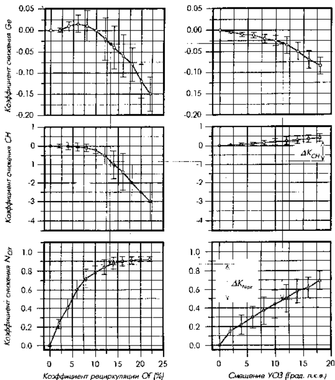
Рис. 6.5.5 Сравнение эффективности методов снижения выбросов NO x : ( V_h = 2.3 л) (Слева- при применении рециркуляцией отработавших газов, справа- при управлении YCO 3 )
